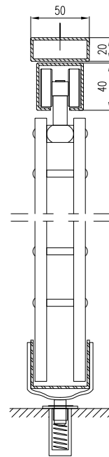
zij aanzicht standaard uitvoering
