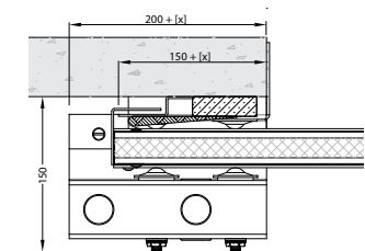
Horizontale doorsnede sluitzijde
