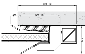
Horizontale doorsnede aanslagzijde
