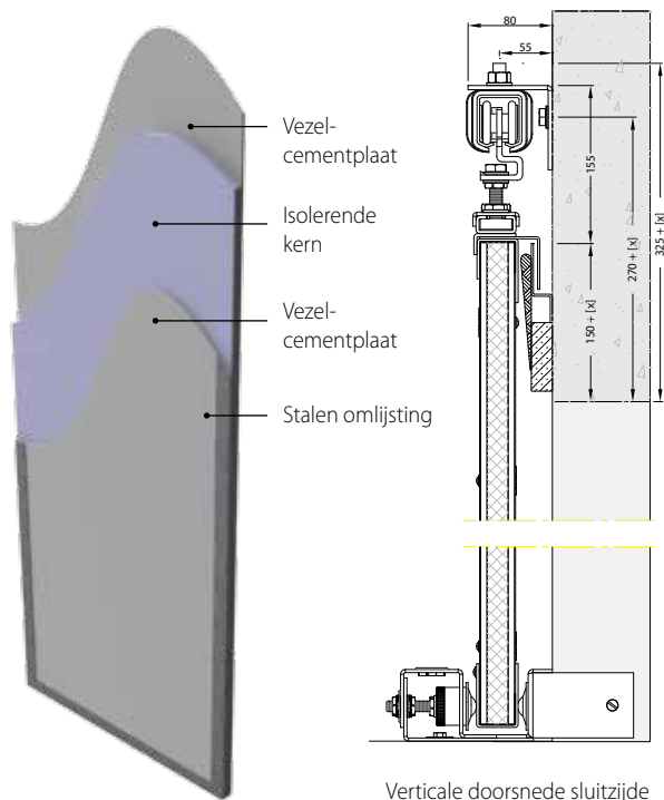
Verticale doorsnede sluitzijde
