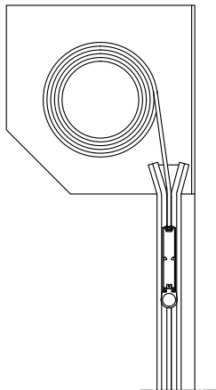
Zijaanzicht oprolmechanisme
